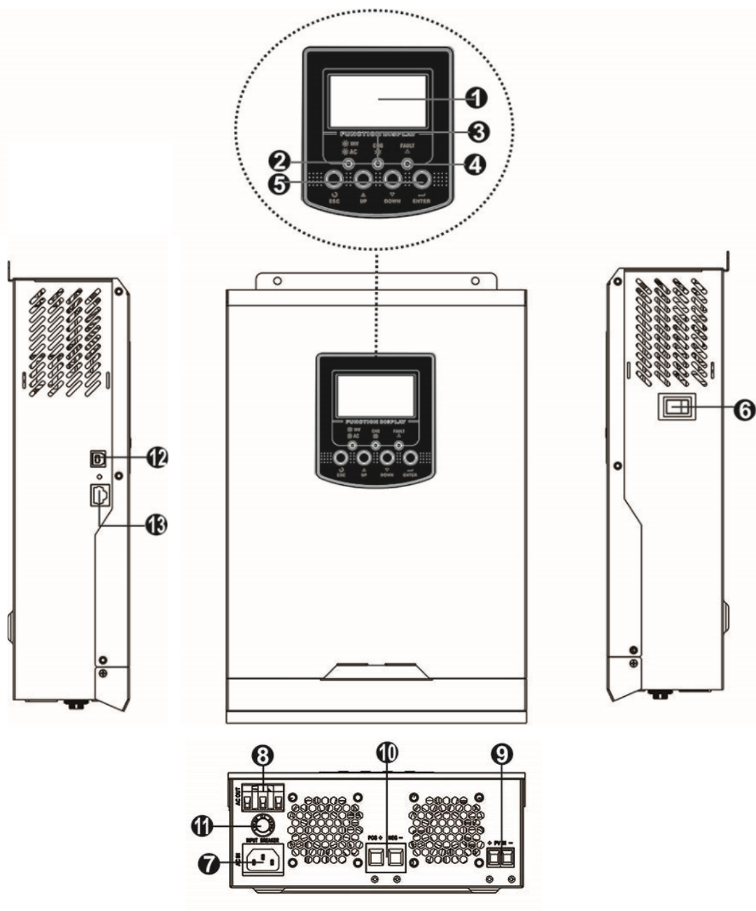
Рисунок 2. Инвертор SMARTWATT ECO 1K 12V PWM.
