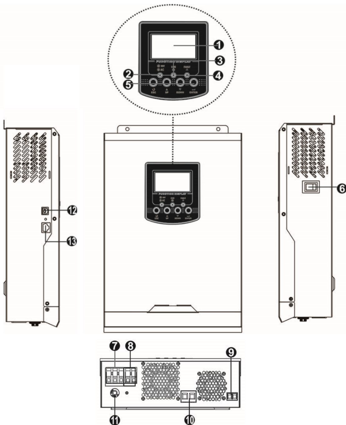
Рисунок 4. Инверторы SMARTWATT ECO 3K 24V PWM и SMARTWATT ECO 3K 24V MPPT
