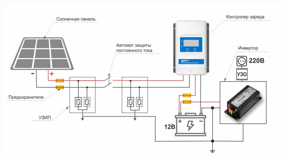
Рисунок 1 Схема подключения преобразователя серии ИС2 к системам альтернативной энергетики
