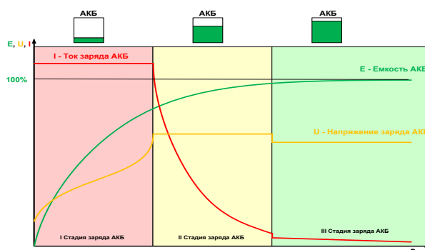
Рисунок 4.5.1 (Процесс заряда аккумуляторной батареи).
